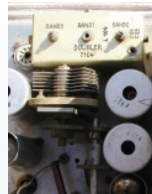
Bandfilter-TX gebaut 1963
