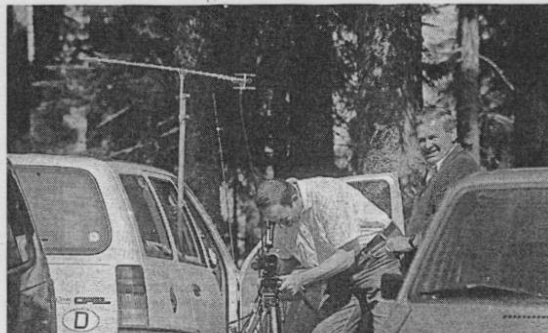
Videokamera und Sendeantenne am Stöcklewaldturm: Der Anfang einer Übermittlungsstrecke für Fernsehbilder. Bilder: Müller
