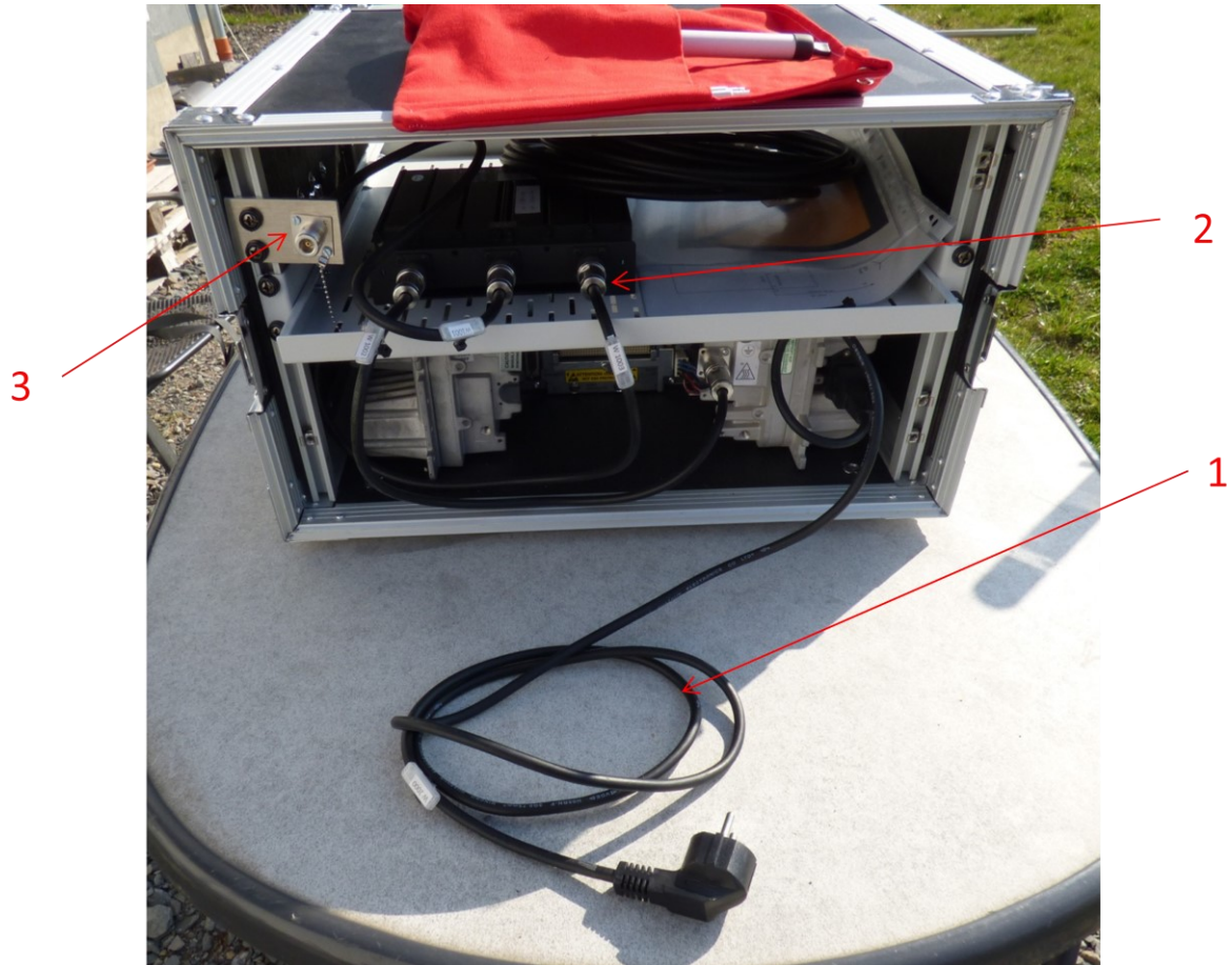
Abbildung 2: Rückseite des Relais
