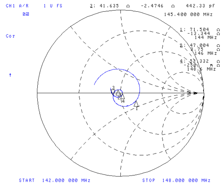
GP-93N Smith Diagramm
