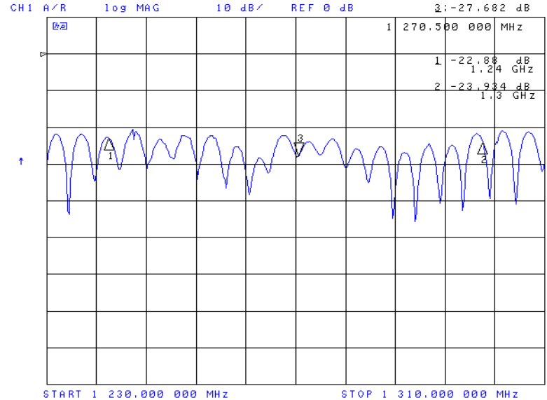
GP-93N 23cm S11
