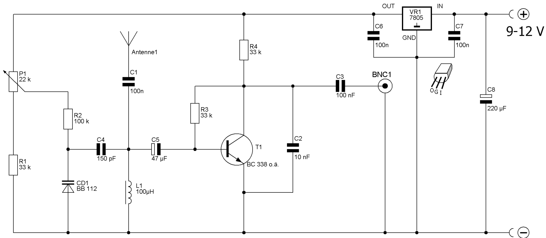
MW/KW-RX mit Varicap
