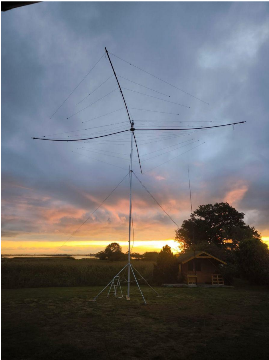
Spider Beam und Vertikal mit Radials
