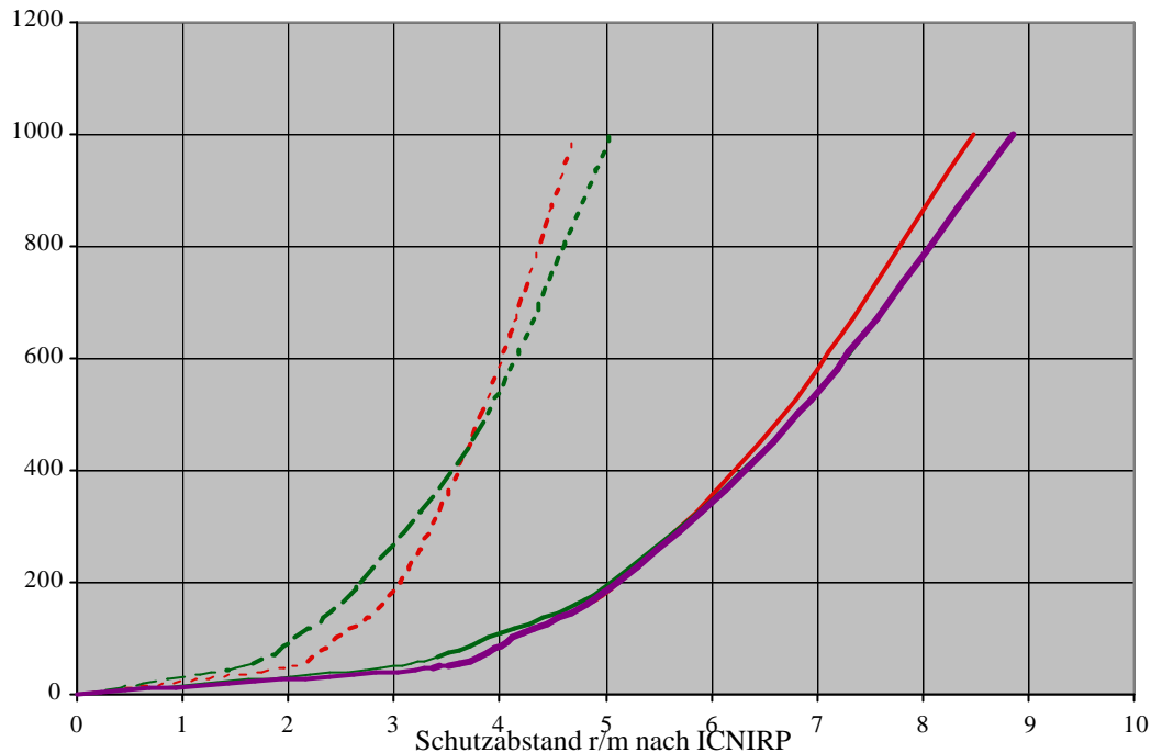
Bild 11.1 Gefittete Schutzabstandskurve r_{S \text{ PERS(BEMFV)}} (rechte dicke Kurve) für die Grundplane 4-BTV bei 7,05 MHz.
