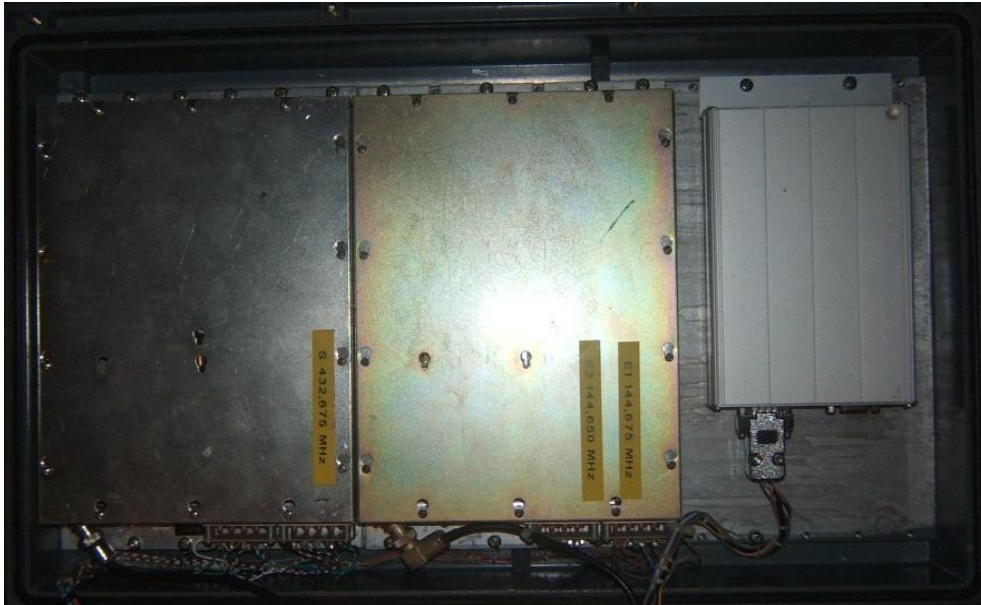
Transponder 2 m - 70 cm Transponder Innenansicht Alles eingebaut in zwei Gehäusehalbschale. (ehemals ein Stornofunkgerät)
