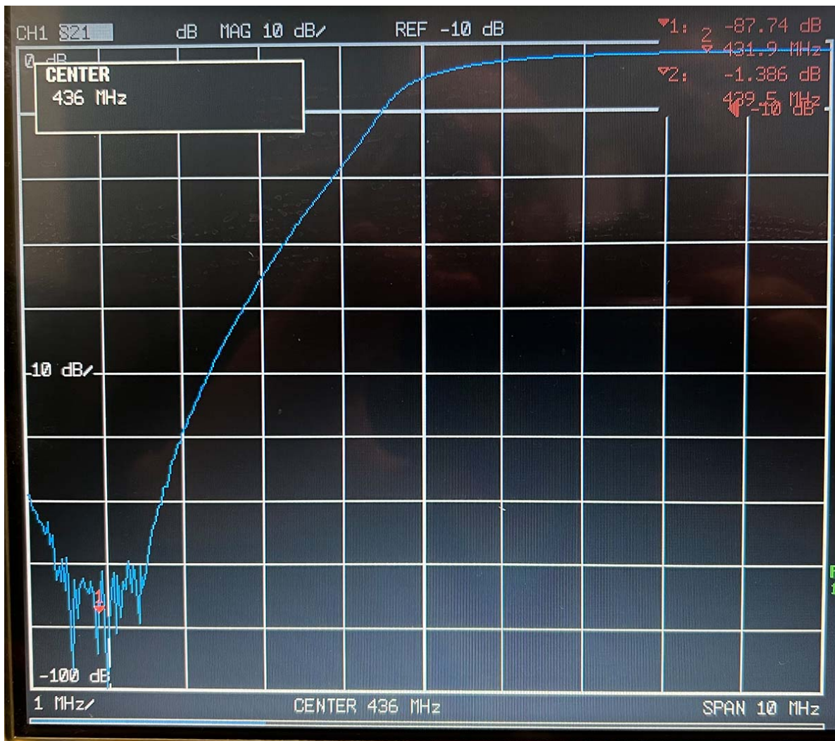
Abbildung 1: TX-Zweig, 439,4875 MHz nach Neuabgleich
