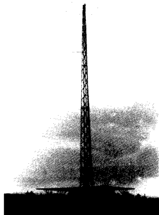
Abb. 3. Gittermast von LXÖRL; auf der Spitze 3-Element-full-size-Beam für 40 m (drehbar), darunter 2-Element-full-size-Draht-Beam für 80 m, umschaltbar in Ost-West-Richtung
